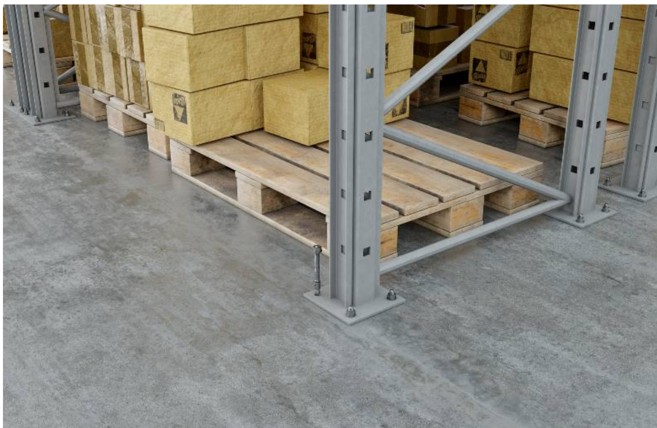
LE-ZNA4 kotwa mechaniczna ocynkowana plus klips ze stali nierdzewnej A4
